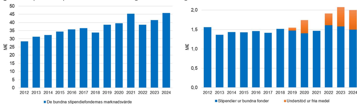
Figur 2. Stipendiekapitalets värdeutveckling samt utdelningen av understöd
